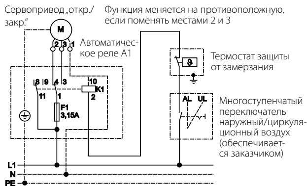
Схема соединений в сочетании с устройством TLH
