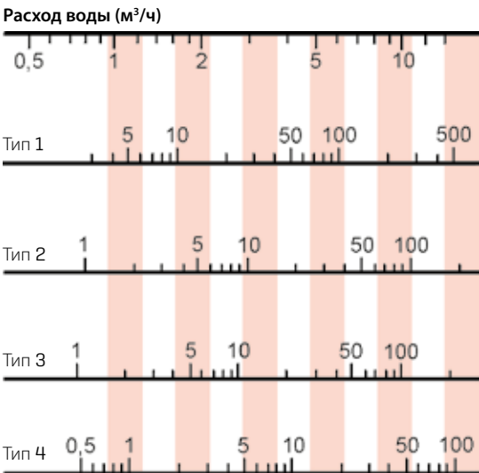
СОПРОТИВЛЕНИЕ ВОДЫ LH-EC / LH 63
