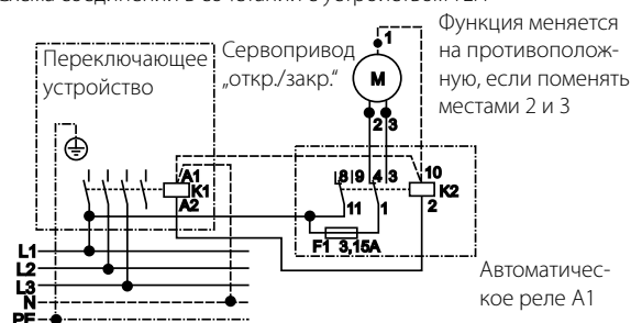
Схема соединений в сочетании с устройством TLH
