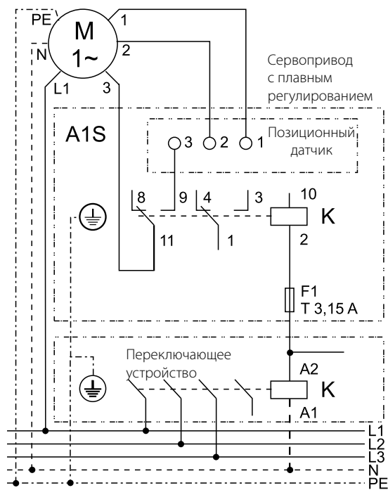
Схема соединений в сочетании с устройством TLH
