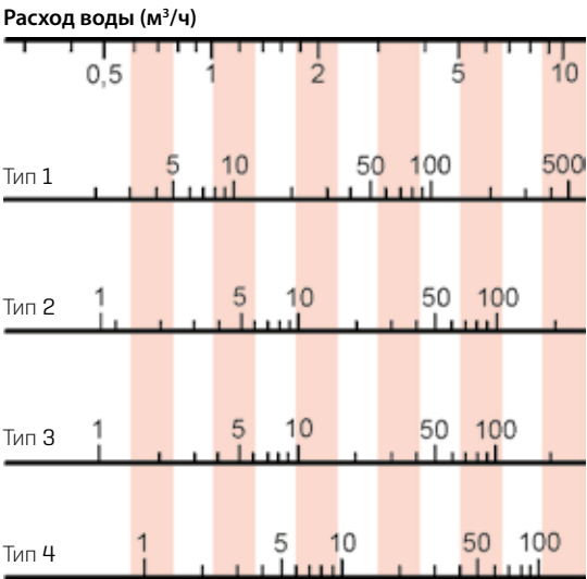
СОПРОТИВЛЕНИЕ ВОДЫ LH-EC / LH 40
